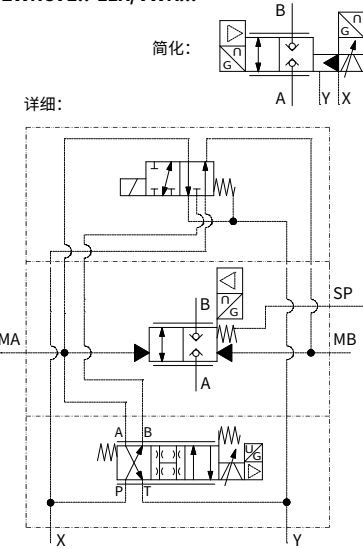
2WRCVE...-L1X/VWK...
