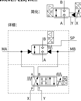
2WRCVE...-L1X/VK...
